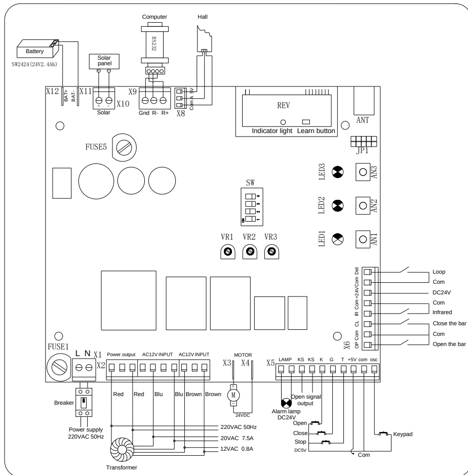
Rys. 9 Tablica rozdzielcza
